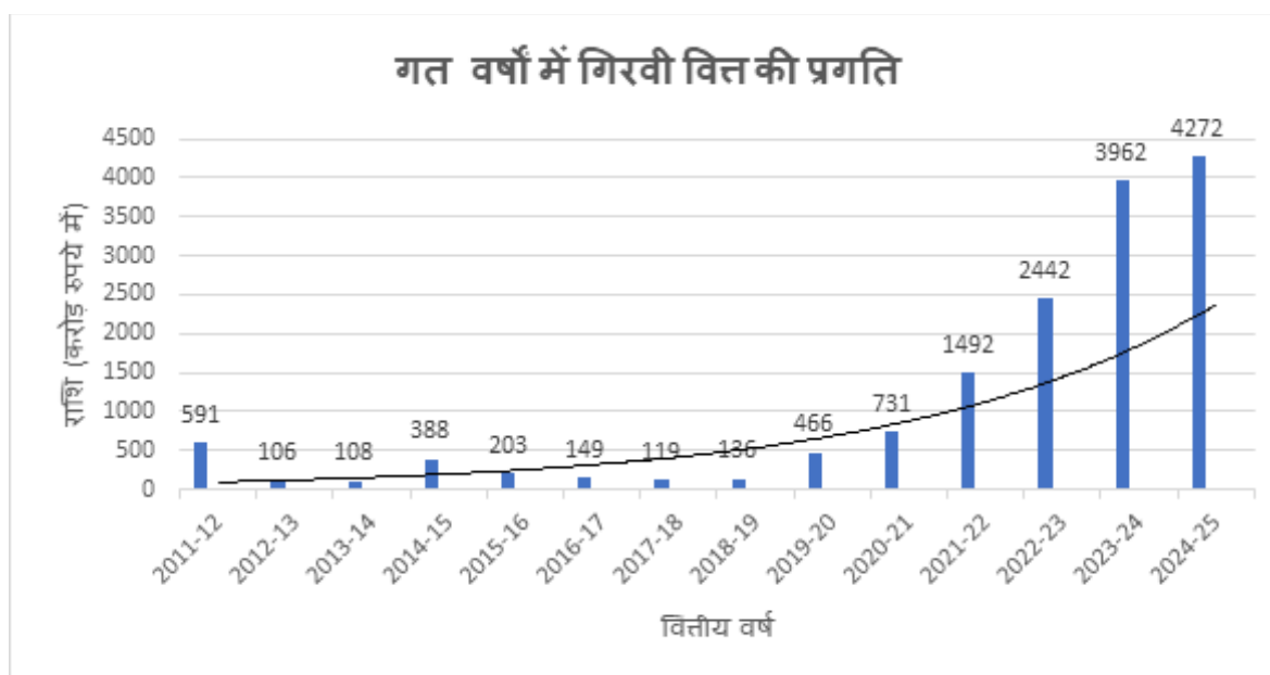
चित्र 4.1
